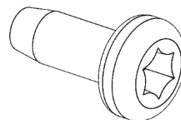
Винт резьбовыдавливающий нерж. M5x12 DIN 7500C T25
